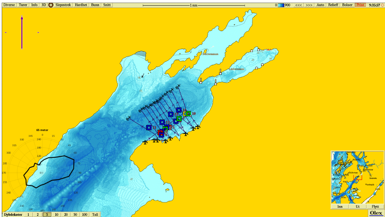
Figur 3: Kartet viser anleggsplassering sammen med B-stasjoner de fire ekstra stasjonene utenfor anleggsramme og fortøyningslinjer. Lilla pil viser orientering av kart, strømse viser vanntransport ( m^3/m^2/døgn ) for hver 15^\circ sektor på 65 meters dyp (spredningsdyp), og gult kryss markerer posisjon for strømmålingene i 2019 ( 65^\circ 21.062'N 12^\circ 26.038'\text{Ø} ; Sivertsen, 2019). Målestokk vises øverst i bildet. Kilde: Olex. Kartdatum WGS84.
